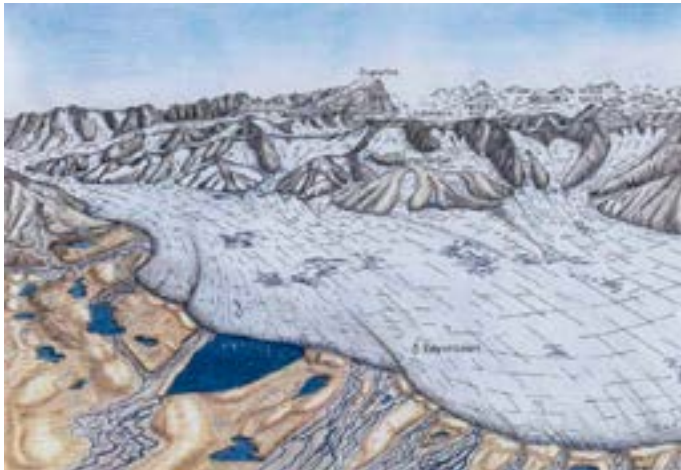
Eiszeitgletscher über dem Oberland vor ca. 10.000 Jahren
